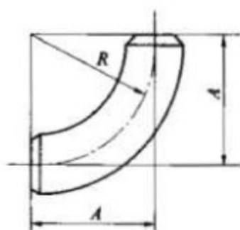
图 B.3 90° 弯头
