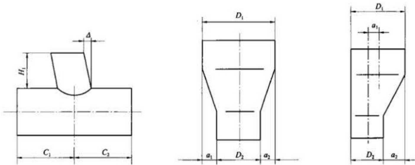
图 E.2 焊接三通支管垂直度示意图
