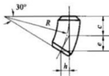
图 B.4 30° 弯头
