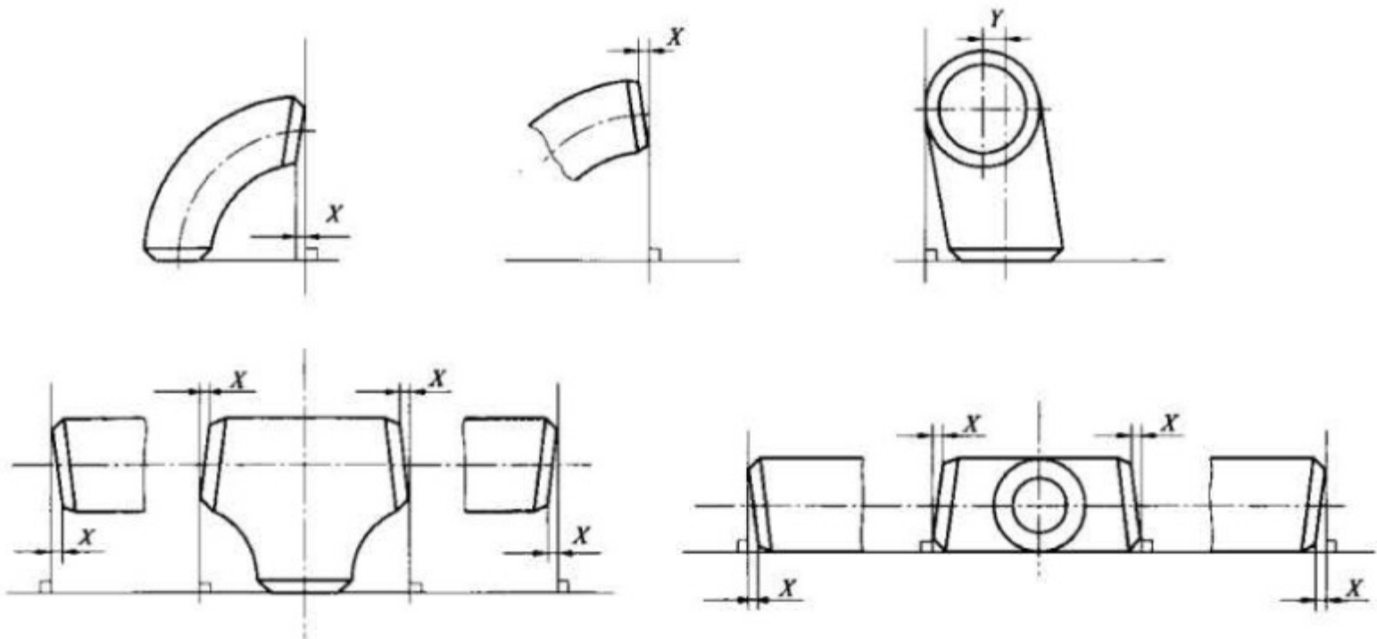
图 E.1 管件形位公差
