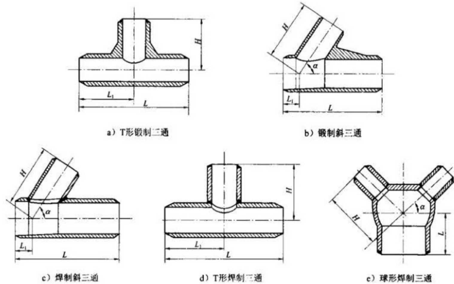
图 D.1 锻制及焊制三通示意图
