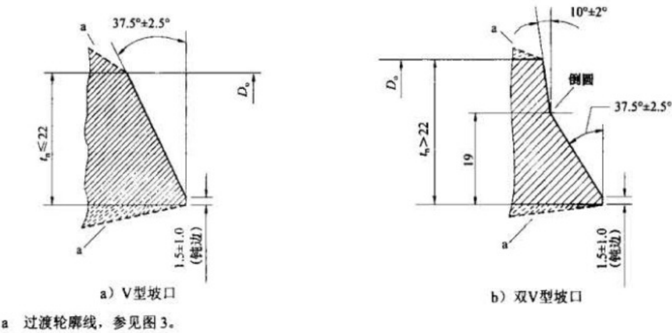
图 2 管件端部坡口形式
