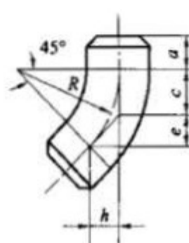
图 B.2 带直段 45° 弯头
