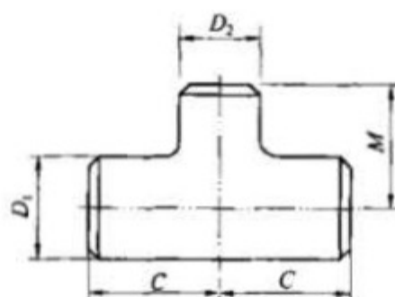
图 B.5 热压三通示意图
