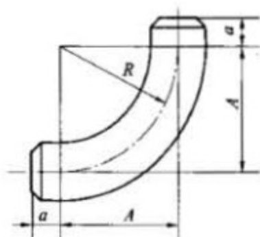
图 B.1 带直段 90° 弯头
