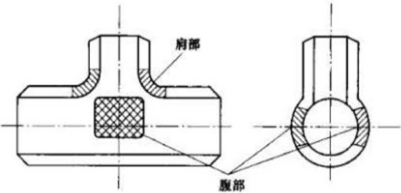
图 1 三通肩部和腹部
